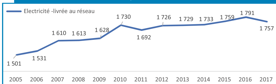
4 Consommation d'électricité de 2005 à 2017, en GWh
