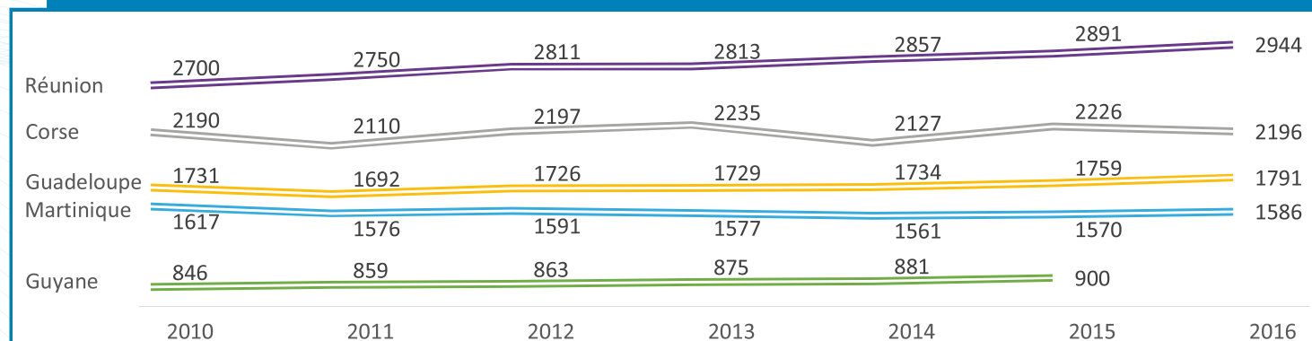
5 Production d'électricité dans les ZNI en GWh
