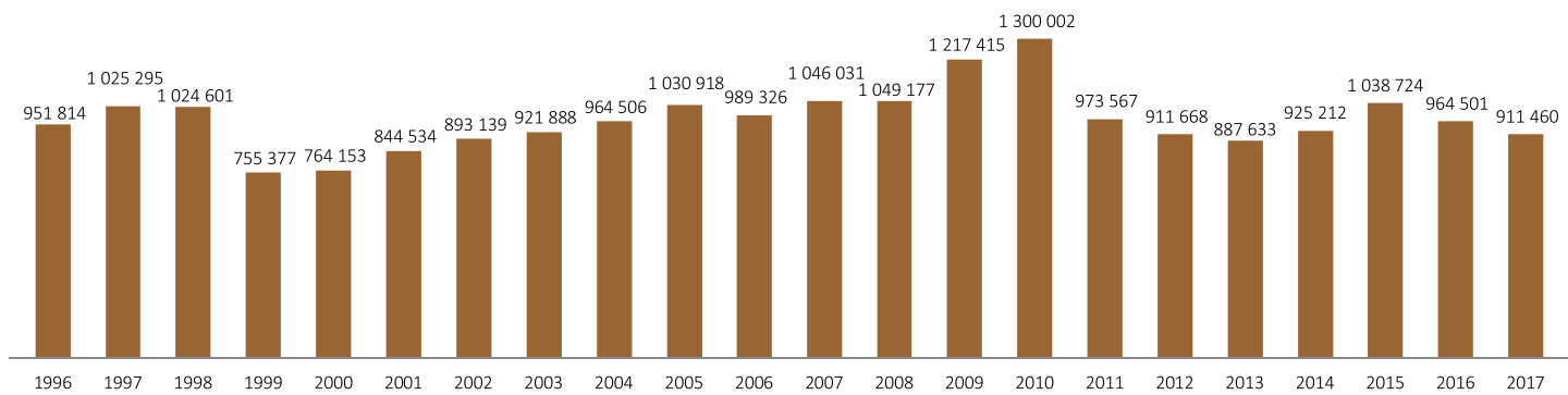
22 Production électrique à partir de produits pétroliers, en MWh
