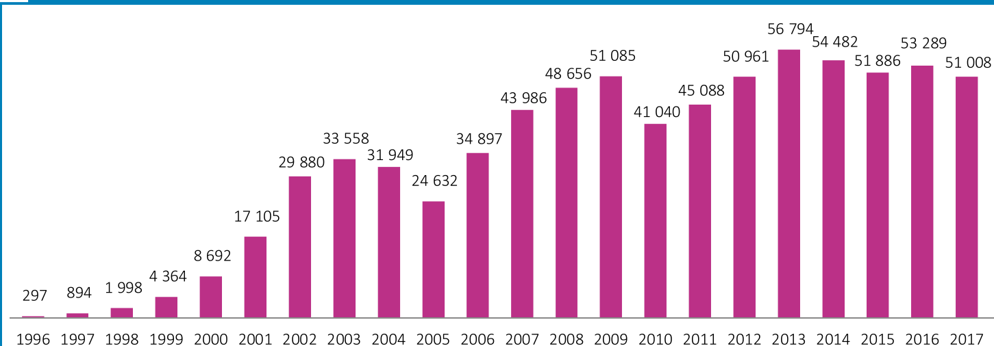
28 Production d'électricité à partir d'énergie éolienne depuis 1996, en MWh
