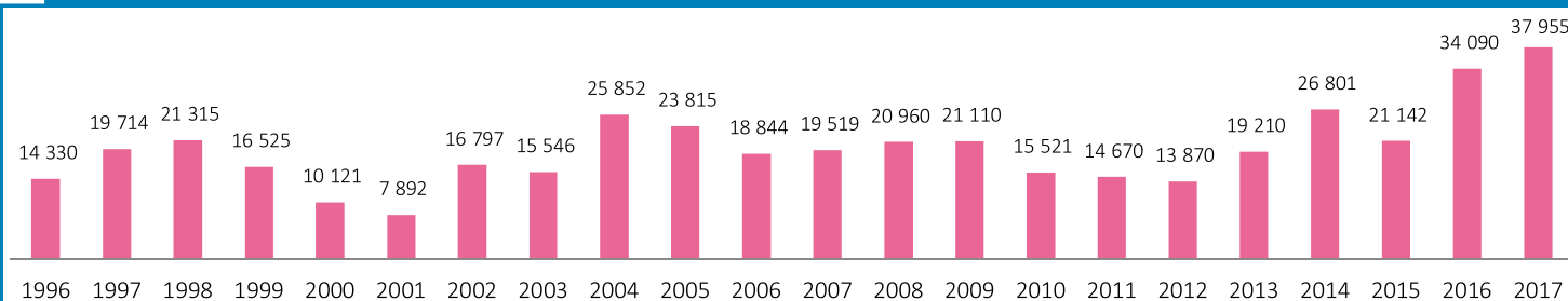
26 Production électrique à partir de ressources hydrauliques depuis 1996, en MWh
