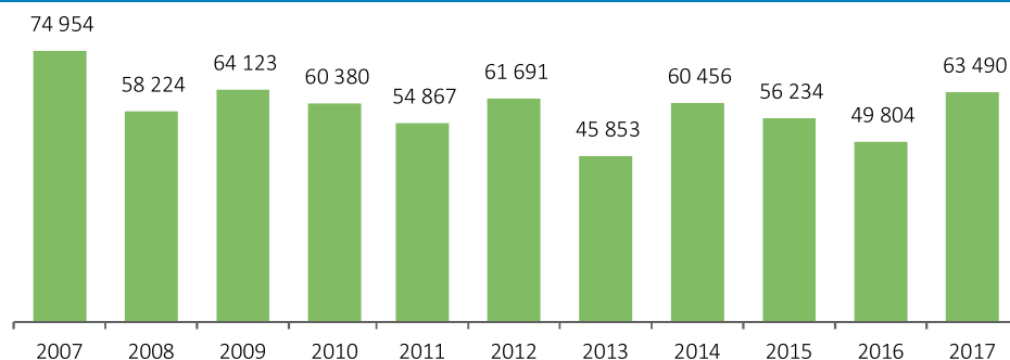
24 Production électrique à partir de bagasse depuis 2007 en MWh
