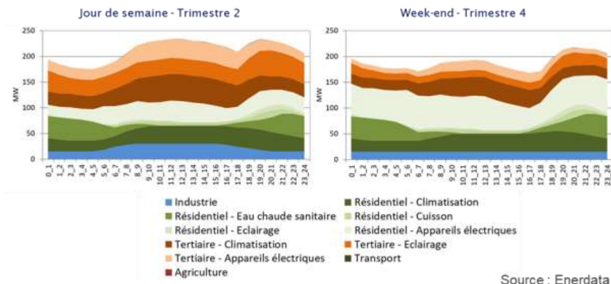
Figure 6 – Résultats de la reconstitution de la courbe de charge journalière pour un jour de semaine au trimestre 2 et pour un week-end du trimestre 4
