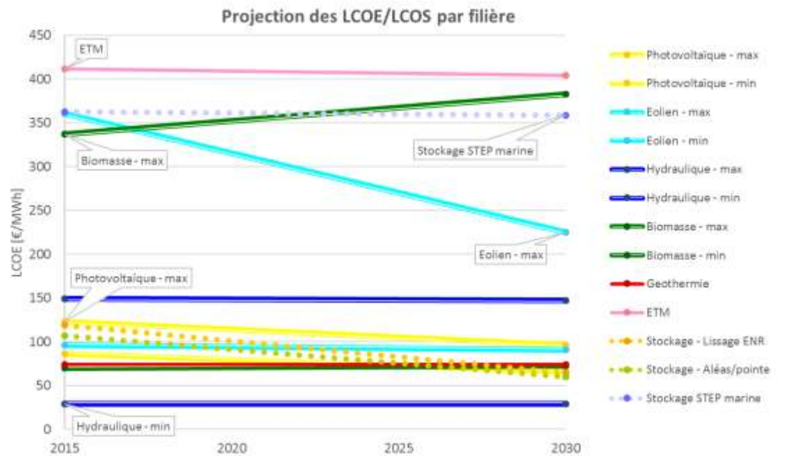
Figure 3 – Projection des LCOE et LCOS moyens sur l'île de la Guadeloupe selon les technologies
