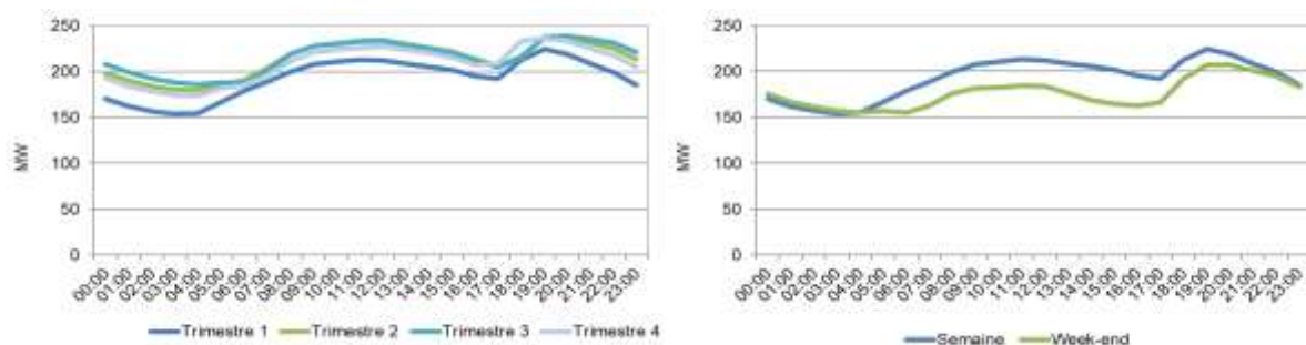
Figure 5 – Courbes de charge 2015 : a) selon le trimestre (jour de semaine) – b) selon le type de jour (trimestre 1) Source : EDF, traitement Enerdata
