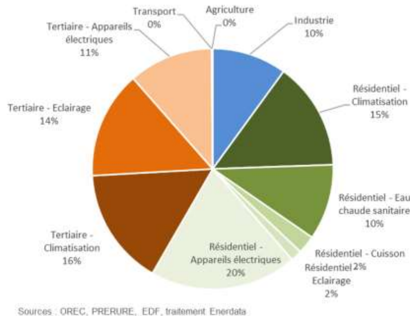
Figure 4 – Reconstitution de la demande d'électricité de la Guadeloupe par secteur et par usage en 2015
