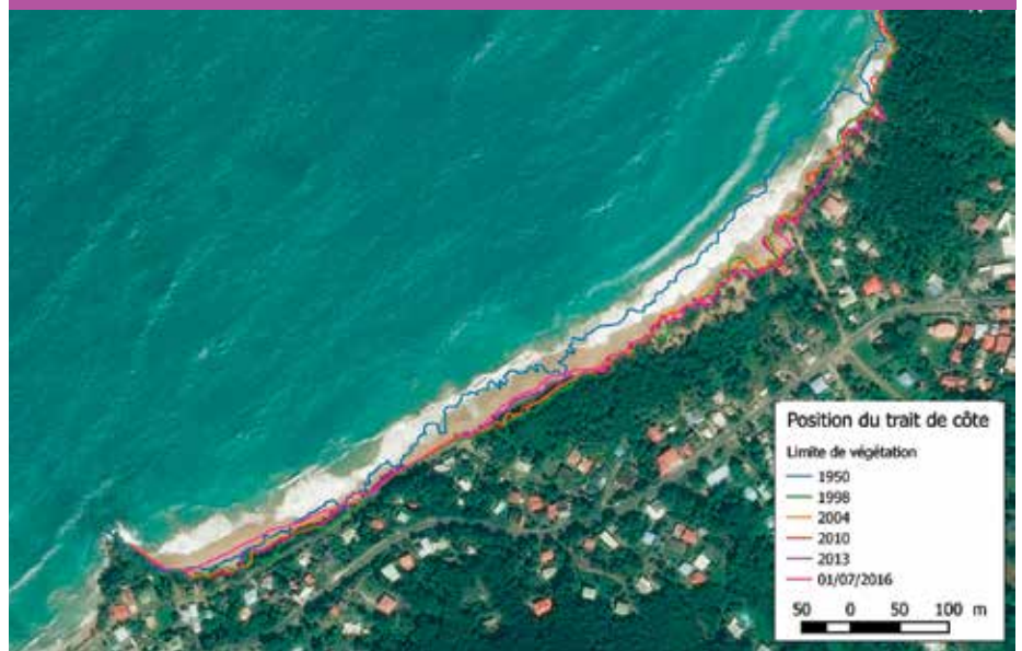
Carte 1 représentative de la variation du traits de côte correspondant à la limite de végétation entre 1950 et 2016 (Fond orthophotographique de l'IGN© 2013)
