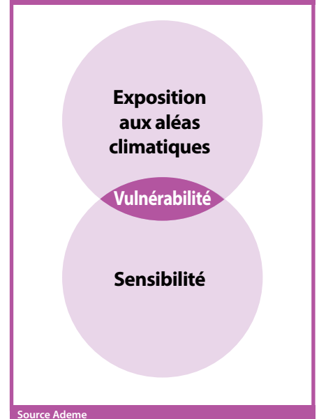
Figure 1 : Lien entre exposition, sensibilité et vulnérabilité
