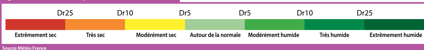
Figure 13 : Standard Précipitation Index
