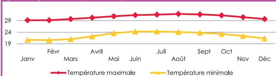
Figure 7 : Diagramme des températures moyennes de la station du Raizet (normales 1981-2010)
