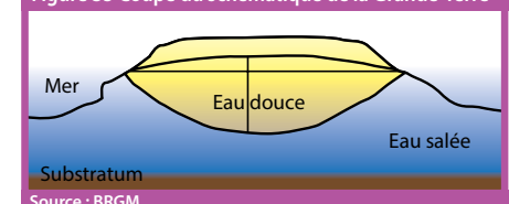
Figure 35 Coupe du schématique de la Grande-Terre
