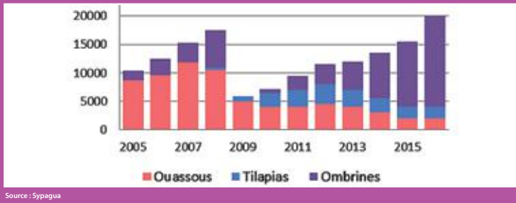
Figure 51 : Evolution de la production en aquaculture en poids vif (en tonnes)
