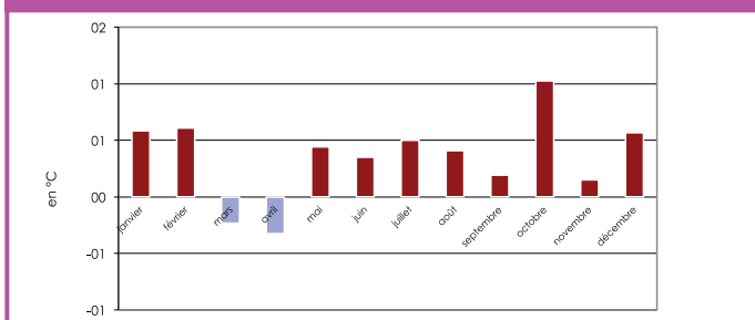
Figure 22 Année 2015 : écart à la moyenne des températures maximales moyennes
