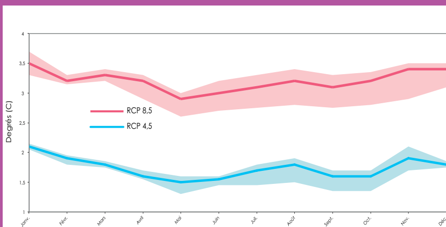
Figure 28 : Projections de températures moyennes maximales pour la période 2090-2099. Ecart par rapport au climat actuel (normale 1981-2010) Source : Météo-France
