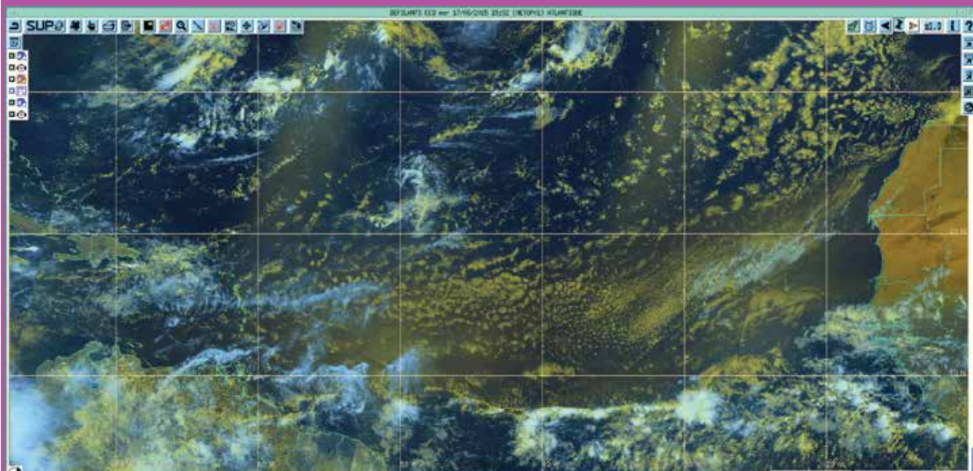
Figure 25 : Composition colorée METOP du 17/06/15 entre 10 :49 et 15 :52 TU : le traitement de différents canaux permet de visualiser la brum4 de sable (teinte jaunâtre qui ternit le bleu de l'océan)
