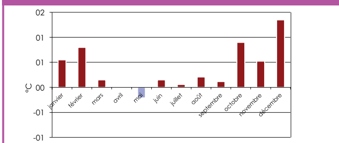
Figure 21 Année 2015 : écart à la moyenne des températures minimales moyennes
